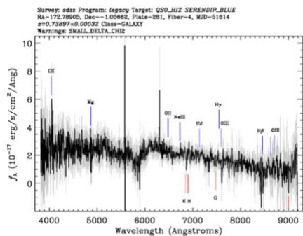
Plate: 281/51614 Fiber: 4
