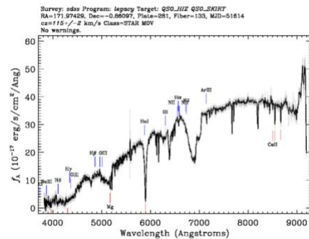
Plate: 281/51614 Fiber: 133
