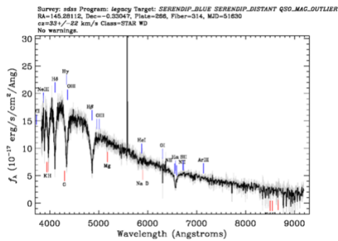
Plate: 266/51630 Fiber: 513
